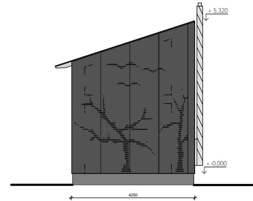
Pohled Východ
