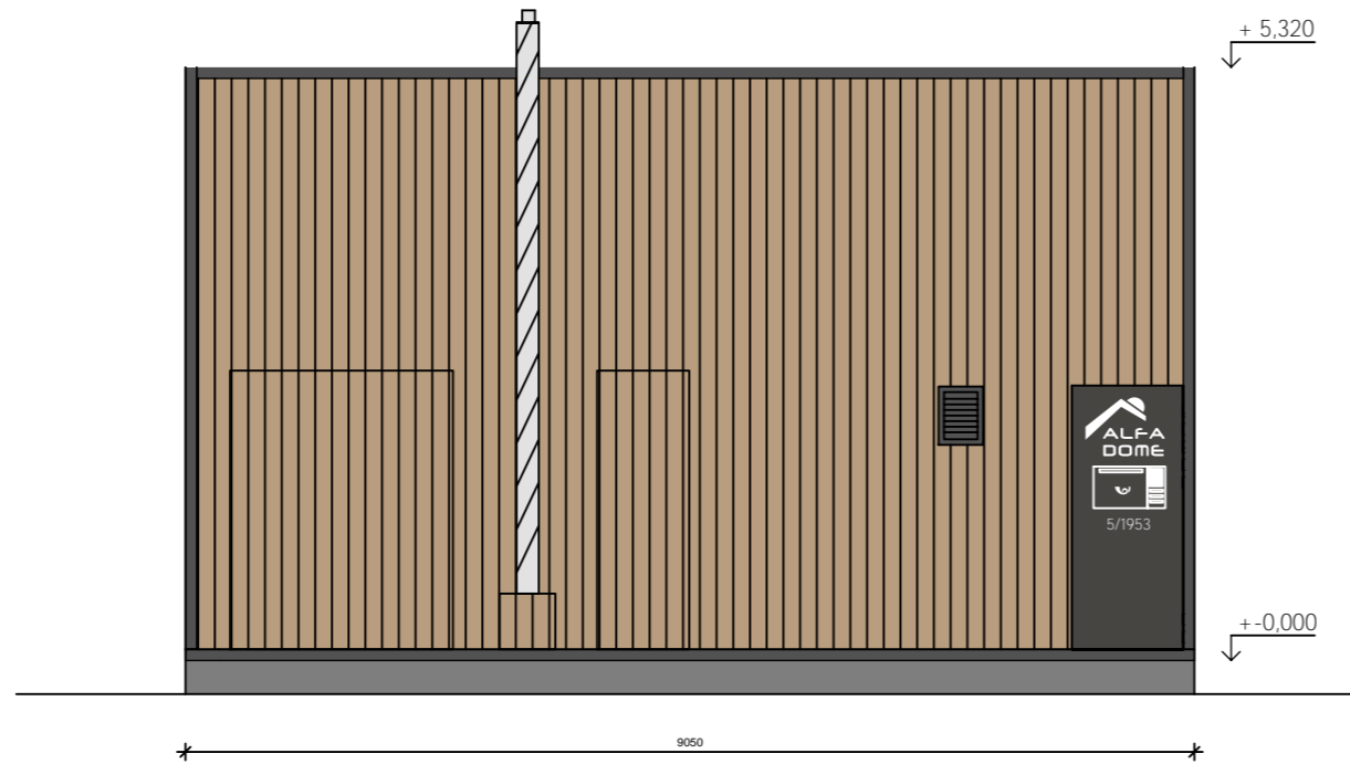
Pohled Sever
